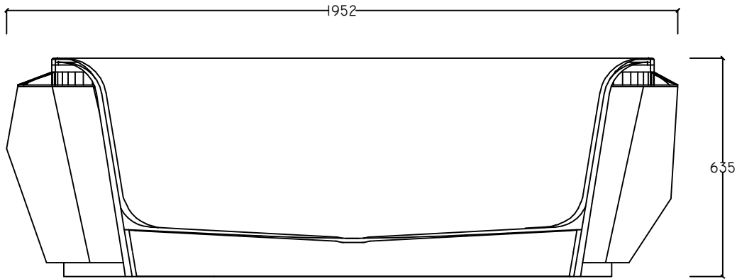
KESİT
